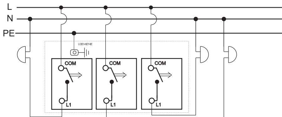
Schemat podłączenia potrójnego łącznika zwiernego.
